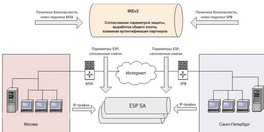
Рис. 1. Архитектура IPsec.
