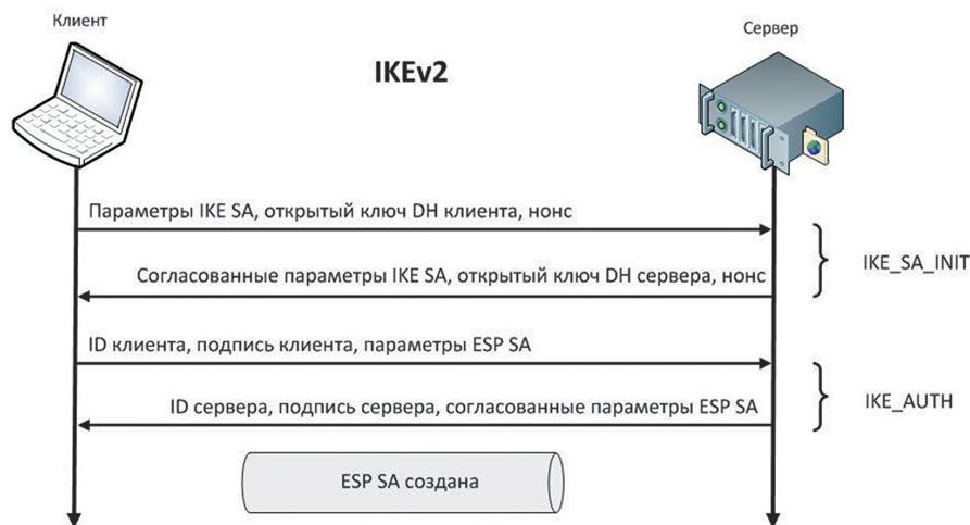
Рис. 2. Создание защищенного соединения в IKEv2.
